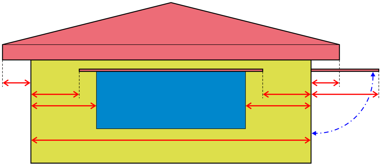
Ansicht Frontseite: Dachüberstand, Verkaufsfenster mit Vordach und geöffnetes Vordach der rechten Seite
